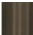
biotite
